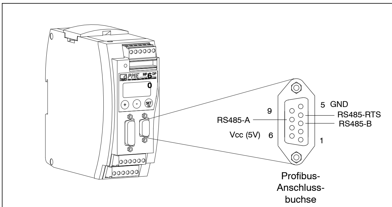
Abb. 4.2: Profibus-Anschluss nach Norm
