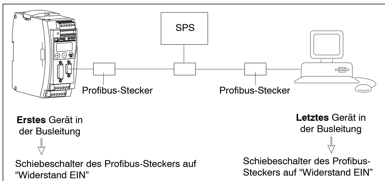
Abb. 3.2: Profibus-Betrieb
