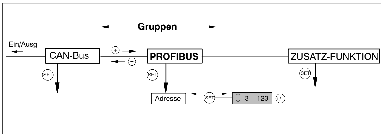
Abb. 5.2: Profibus-Adresse einstellen
