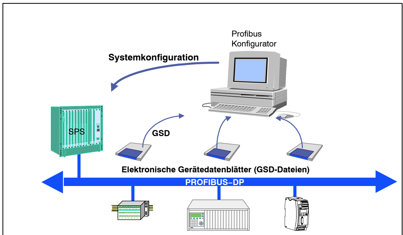
Abb. 2.4: Konfiguration mit GSD-Dateien
